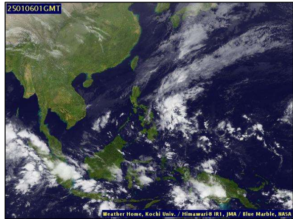
ภาพถ่ายดาวเทียม วันที่ ๖ ม.ค. ๒๕๖๘ เวลา ๐๘.๐๐ น.
